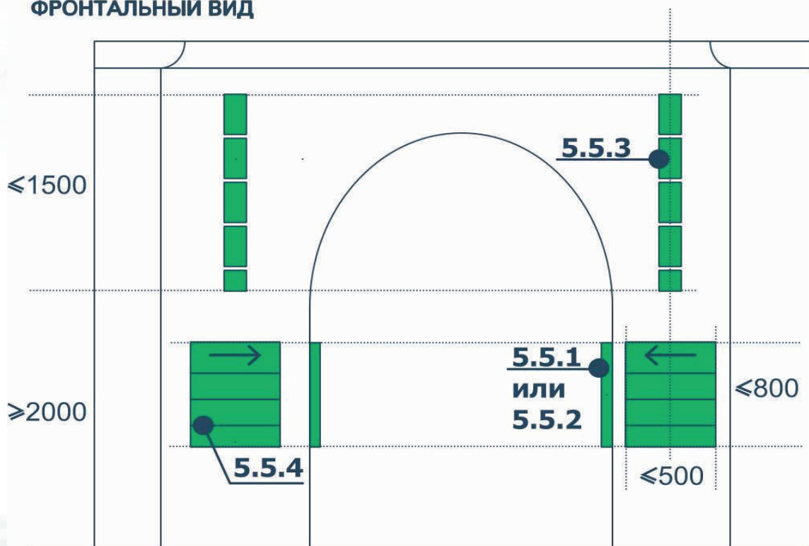
ФРОНТАЛЬНЫЙ ВИД
