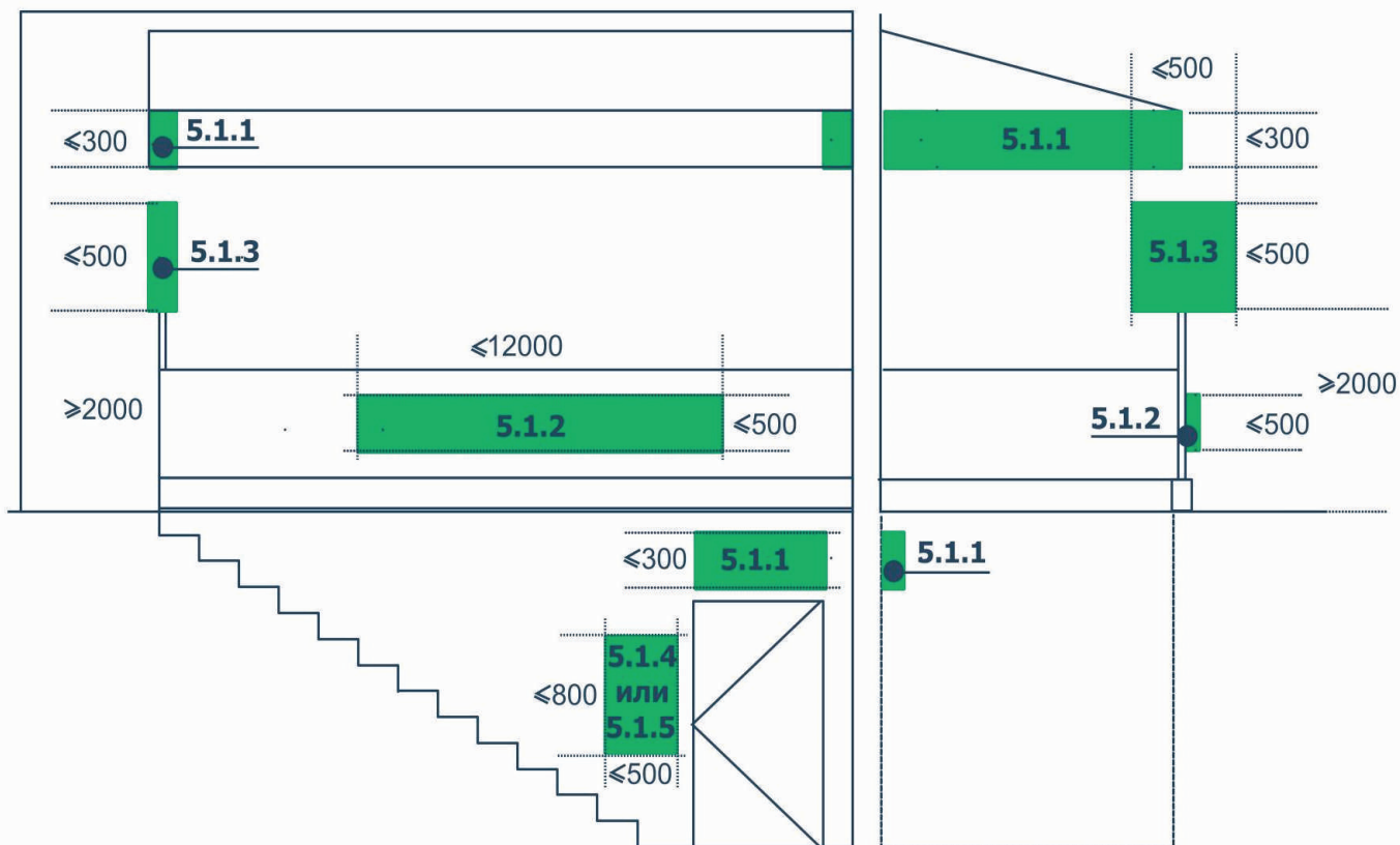
ФРОНТАЛЬНЫЙ ВИД
